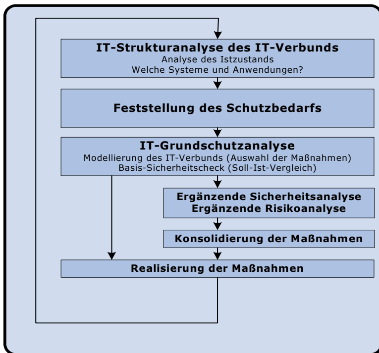
Abbildung 1: IT-Grundschutz-Vorgehensweise
